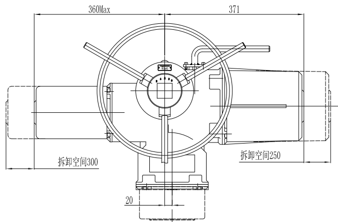
IMC25带HAJBC系列外形及连接尺寸
