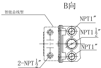
IMC25带HAJBC系列外形及连接尺寸
